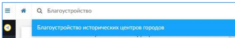
Рисунок 3 – Строка поиска
