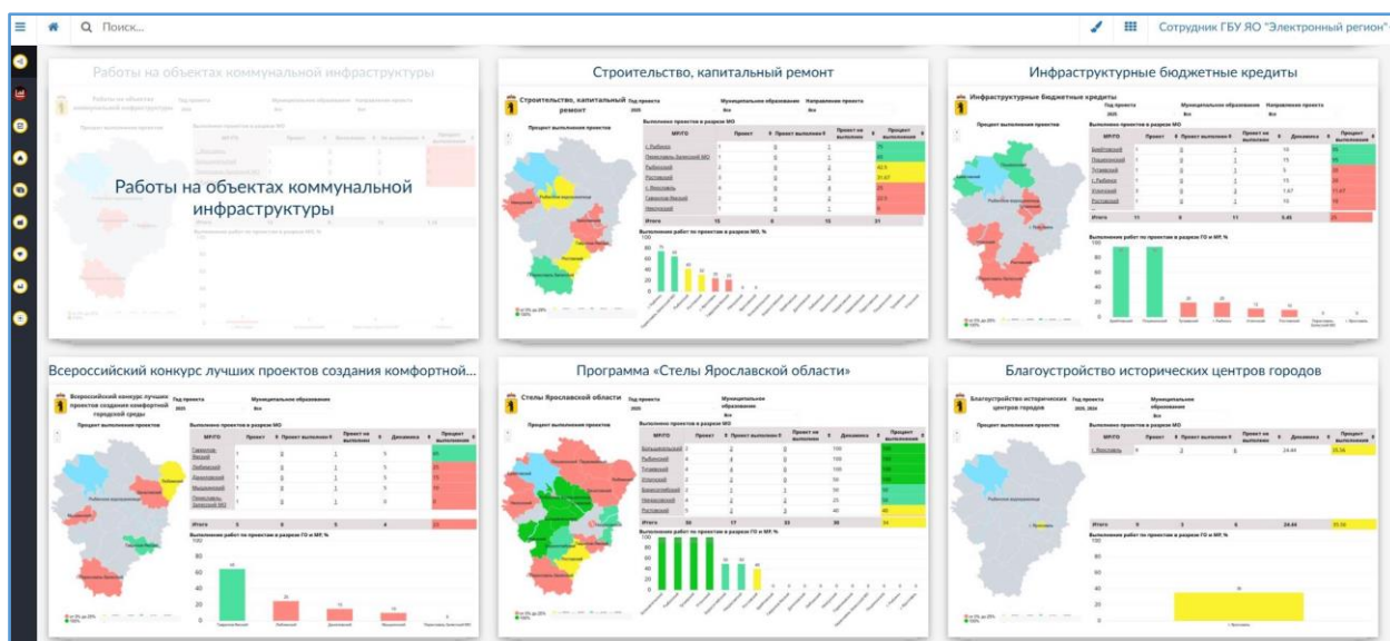
Рисунок 4 – Макеты дашбордов
