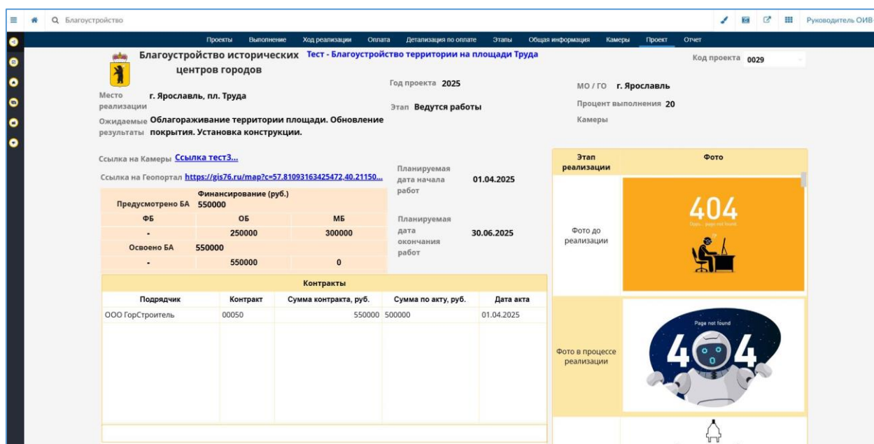
Рисунок 21 – Вкладка «Проект»
