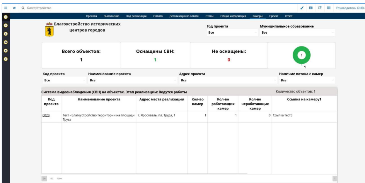
Рисунок 20 – Вкладка «Камеры»
